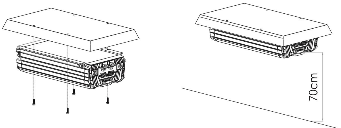
Fig. 8 : Deckenmontage
