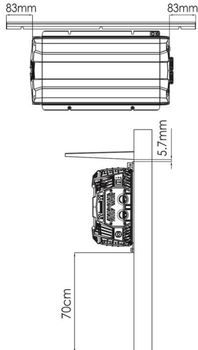
Fig. 7 : Wandhalterung Schritt 2
