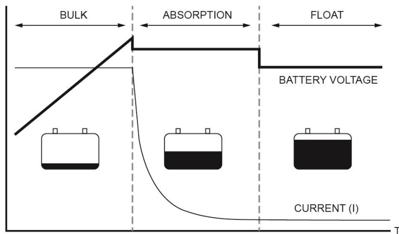
Fig. 9 : dreistufiges Ladesystem
