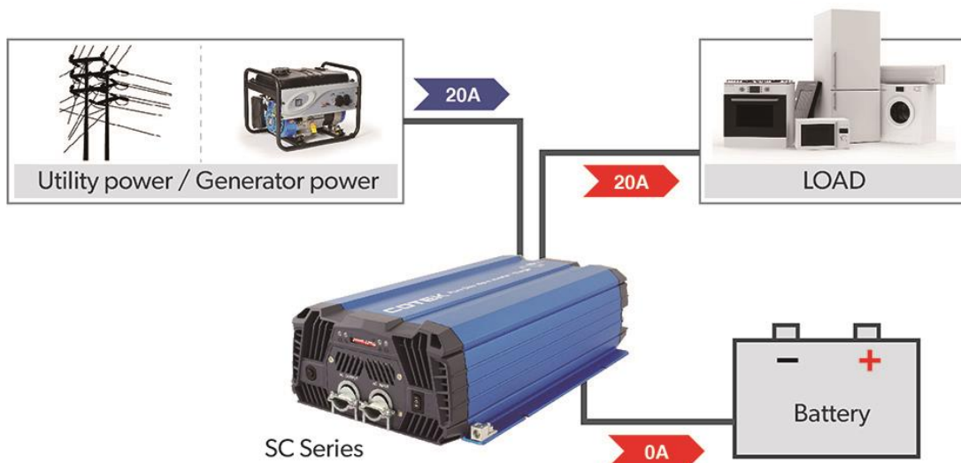
Fig. 15 : Stromaufteilungsfunktion III
