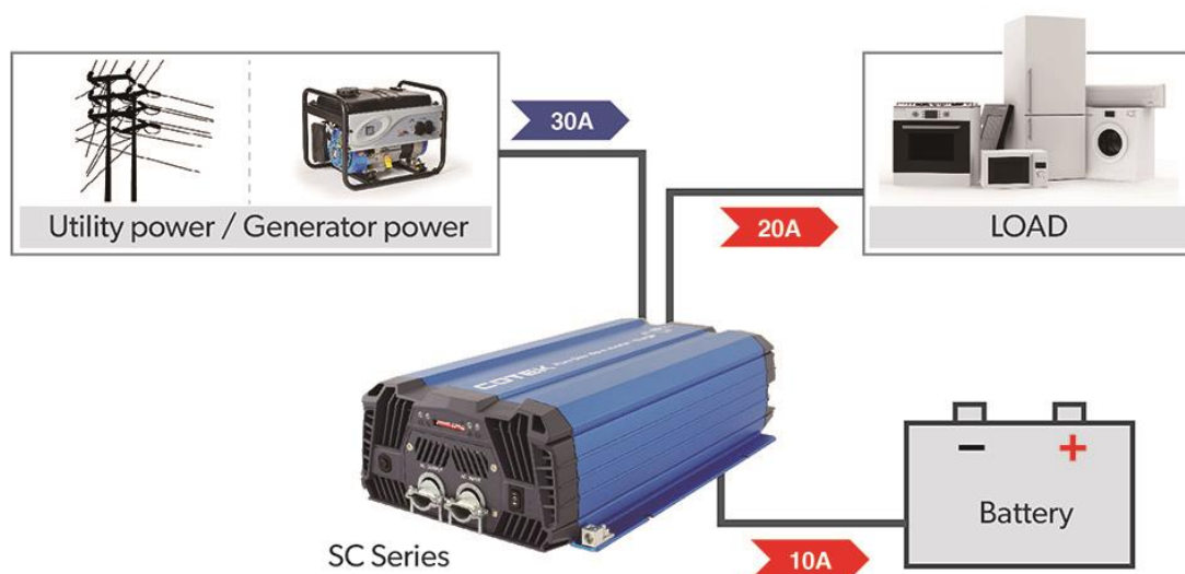
Fig. 14 : Stromaufteilungsfunktion II
