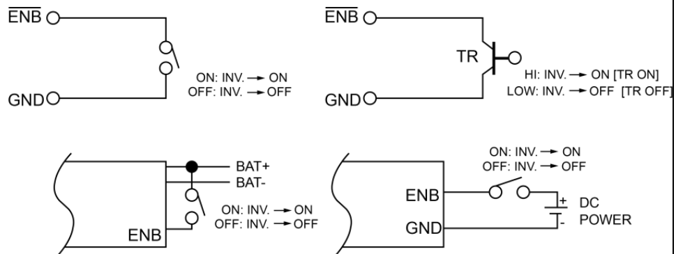
Fig. 8 : Verdrahtung für die Fernbedienung
