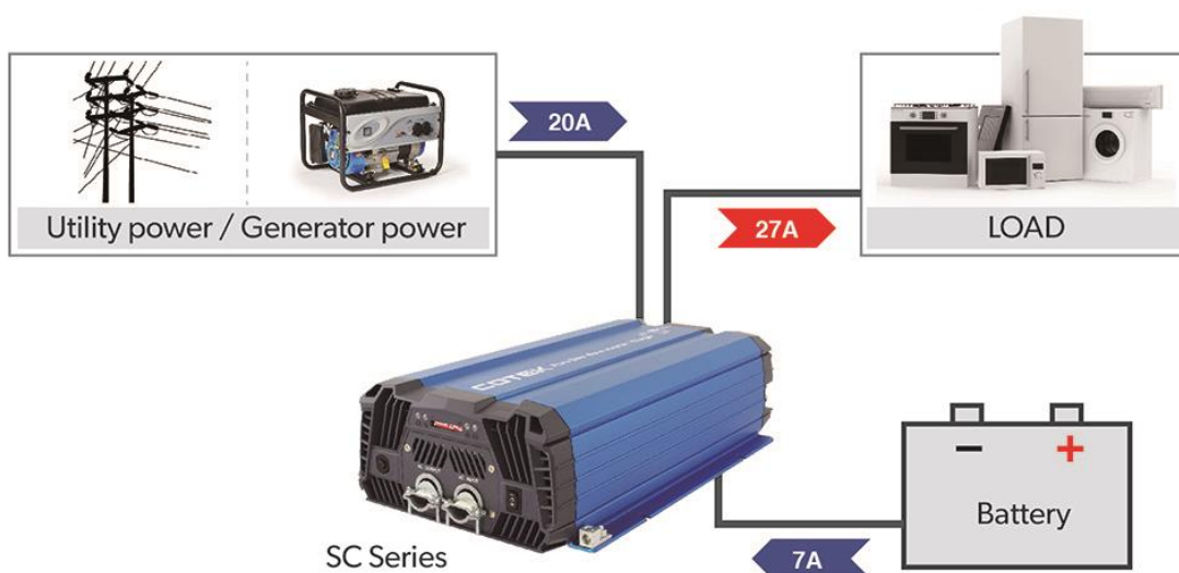
Fig. 16 : Generatorfunktion
