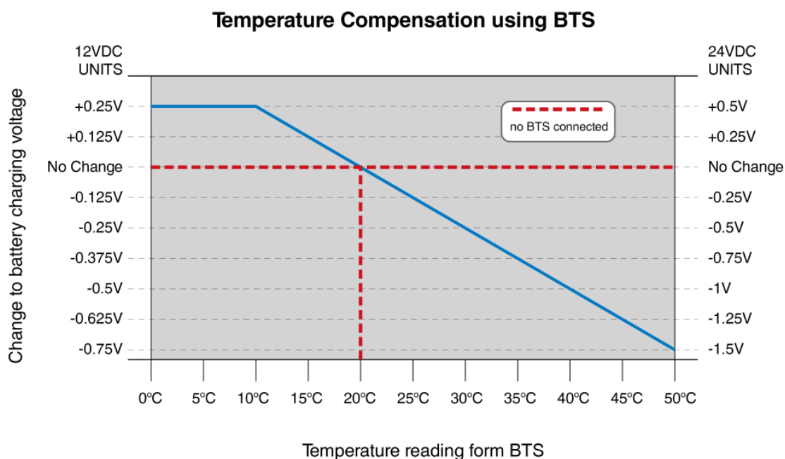
Fig. 10 : Temperaturkompensation mit BTS
