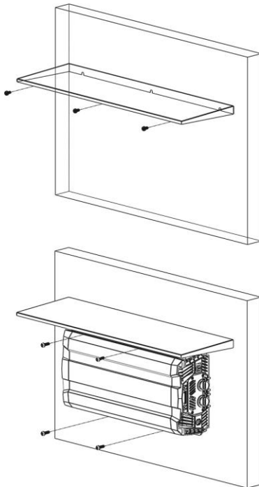
Fig. 6 : Wandhalterung Schritt 1
